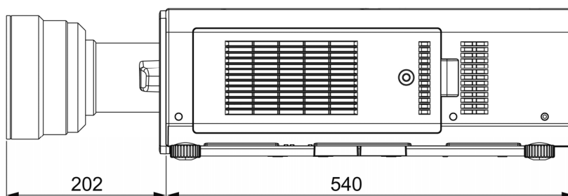
<PT-DZ8700/DS8500/DW8300 に装着した図>
