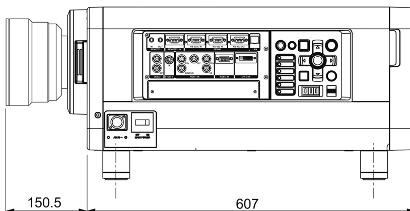
<PT-DZ12000/D12000/DW100,TH-DW10000/D10000 に装着した図>
