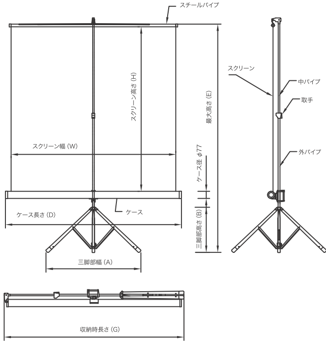
スクリーン・脚部 収納図
