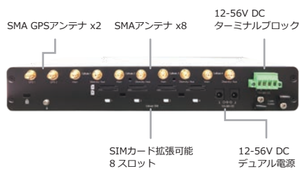
リアパネル
