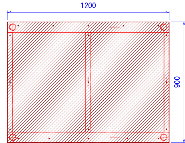
■天板(黒塗装) ■ 1枚 (R01771-02-0-F)
