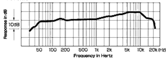
周波数特性
