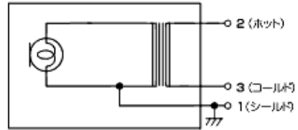
内部結線図
