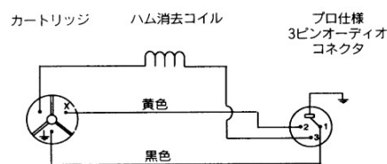
内部接続図
